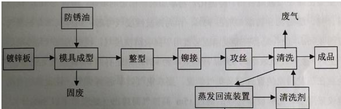
图 3-4 电机零部件工艺流程图
