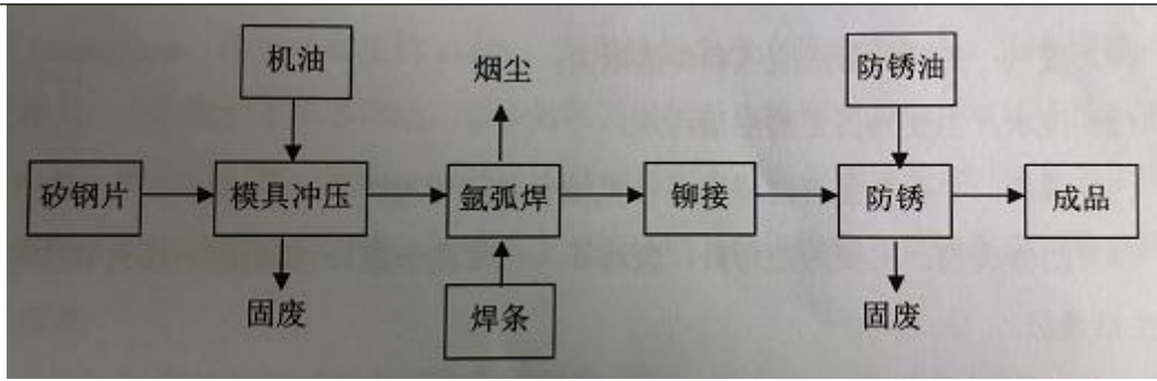
图 3-3 驱动顶级定制冲片工艺流程图
