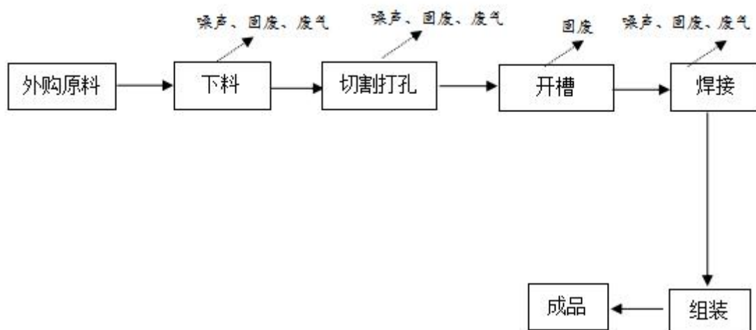
图 2-2 生产工艺流程图
