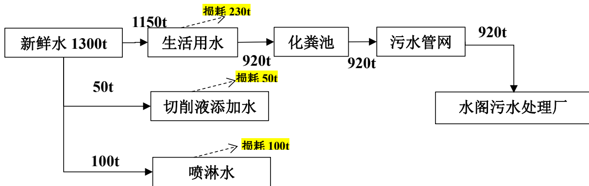
图 2-6 全厂水平衡图
