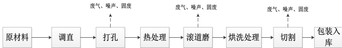
图 2-3 直线导轨生产工艺流程图
