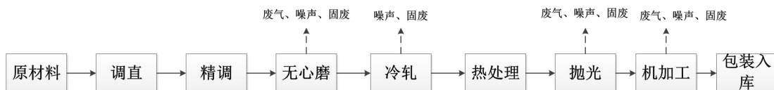
图 2-5 丝杆生产工艺流程图
