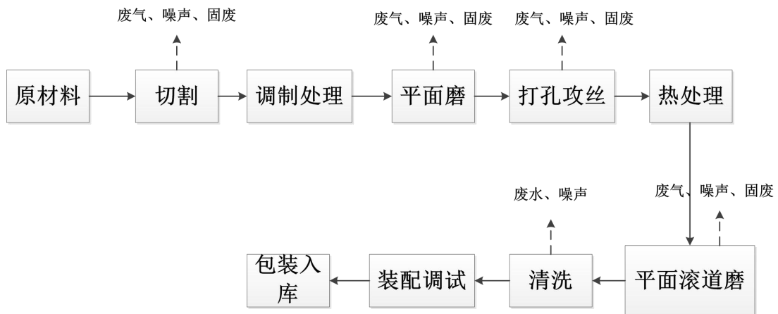
图 2-4 滑块生产工艺流程图
