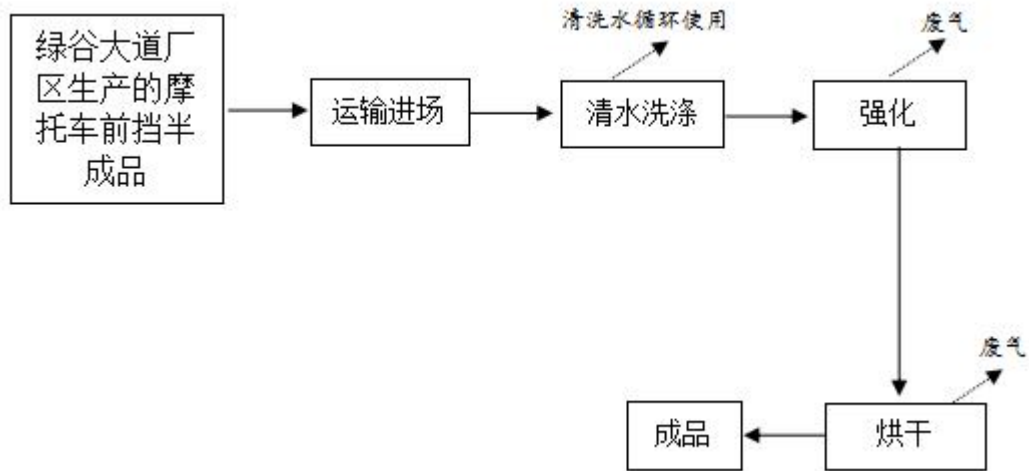
图 3-3 项目工艺流程图
