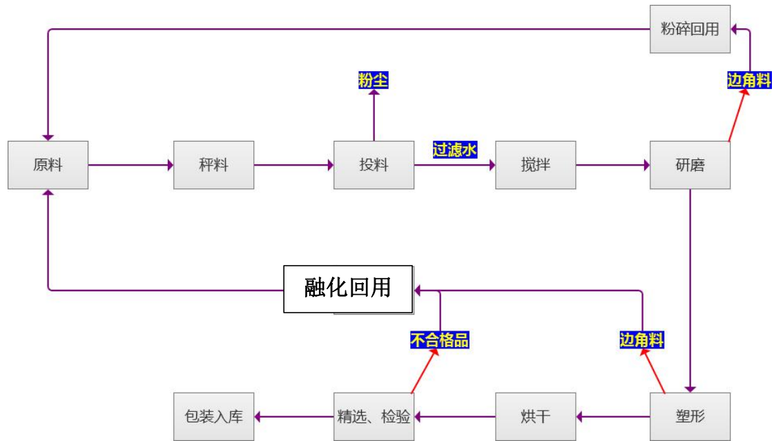
图 3-4 项目蜡笔生产流程图
