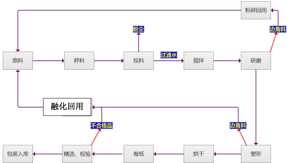
图 3-5 项目油画棒生产流程图
