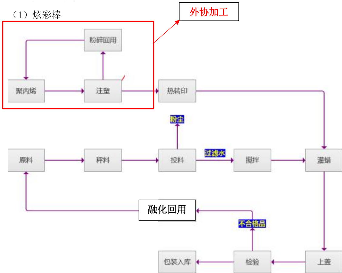
图 3-3 项目炫彩棒生产流程图
